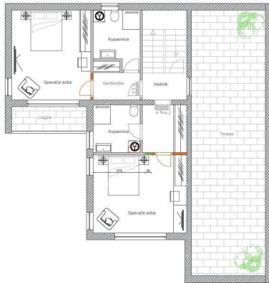
DISPOZICIJA NAMJEŠTAJA - KUĆA A - 1 kat MJ 1:100
