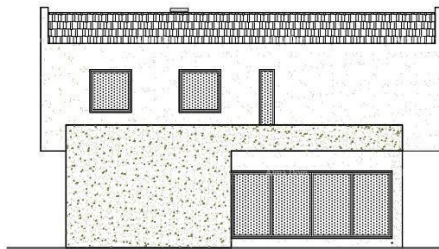
SJEVEROZAPADNO PROČELJE
