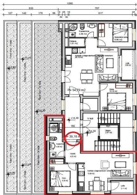
Tlocrt V kata
