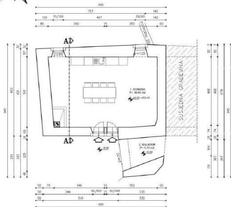
TLOCRT PRIZEMLJA NOVO STANJE M 1:100
