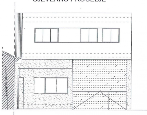
SJEVERNO PROČELJE
