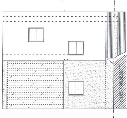
JUŽNO PROČELJE
