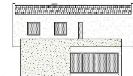
SJEVEROZAPADNO PROČELJE
